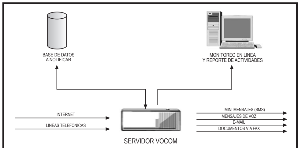
Diagrama Esquemático del funcionamiento del VOCOM NOTIFICADOR
